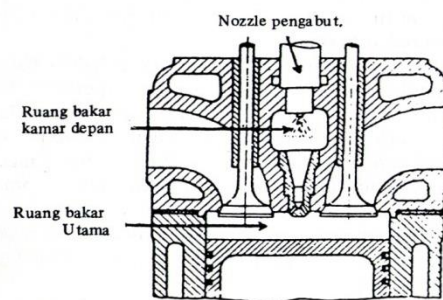
Gambar 2.5. Ruang bakar kamar depan
