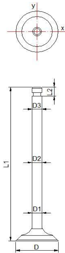
Gambar 3.6. Katup
