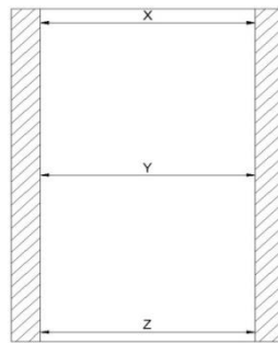
Gambar 3.8. Silinder Liner
