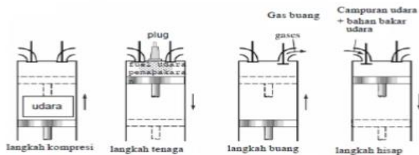
Gambar 2.7. Siklus aktual motor diesel
