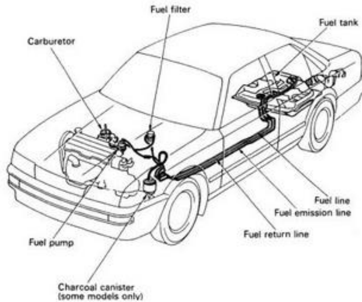
Gambar 3.10. Sistem bahan bakar
