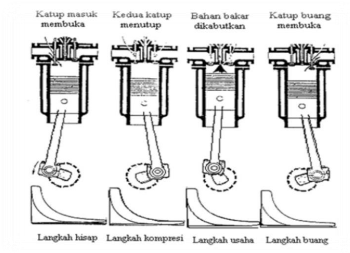
Gambar 2.1. Prinsip kerja motor diesel 4 langkah
