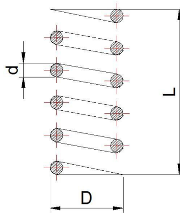
Gambar 3.7. Pegas Katup
