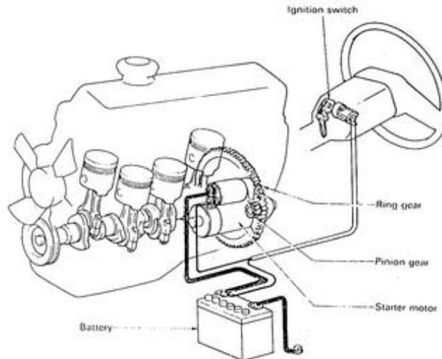
Gambar 3.13. Sistem Starter
