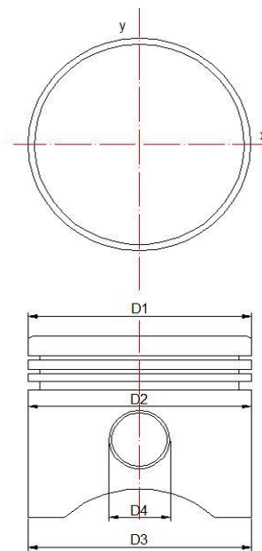
Gambar 3.1. Torak
