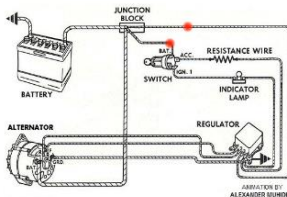
Gambar 3.14. Sistem Pengisian
