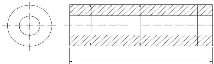
Gambar 3.4. Pena torak
