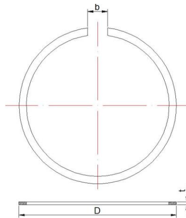
Gambar 3.2. Ring Kompresi
