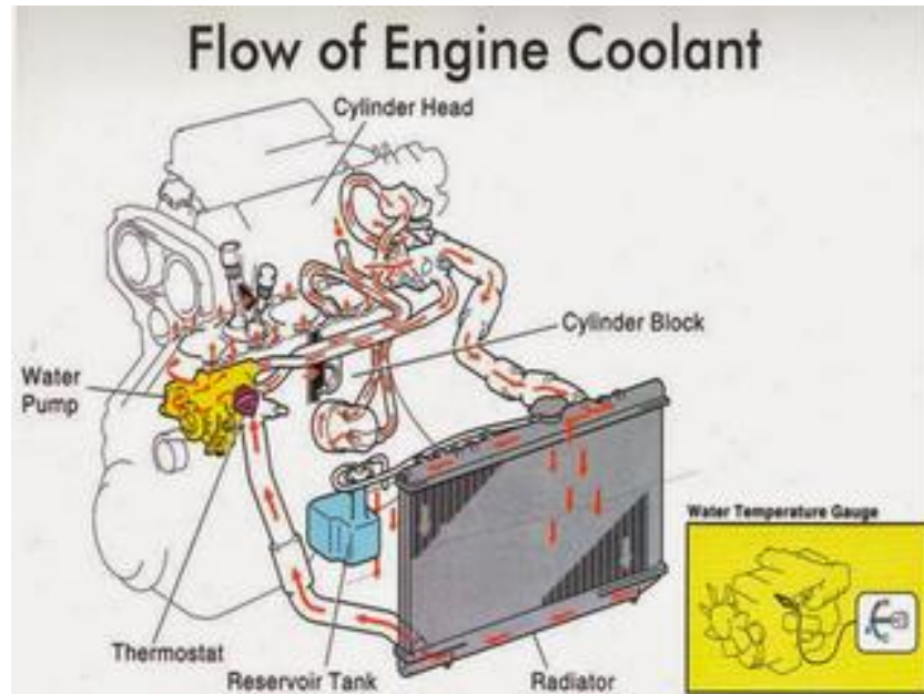
Gambar 3.12. Sistem pendinginan
