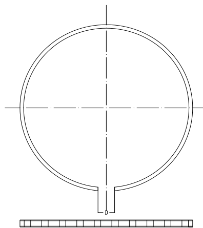
Gambar 3.2. Ring Kompresi
