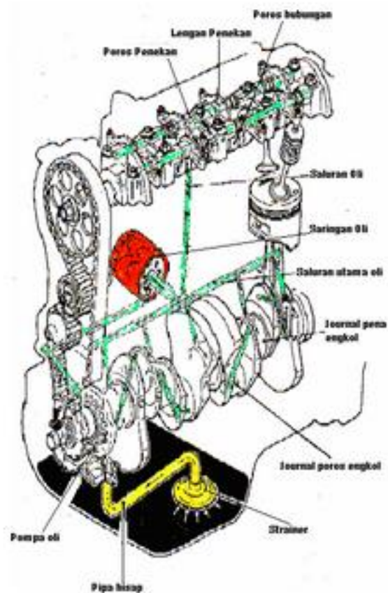
Gambar 3.11. Sistem pelumasan
