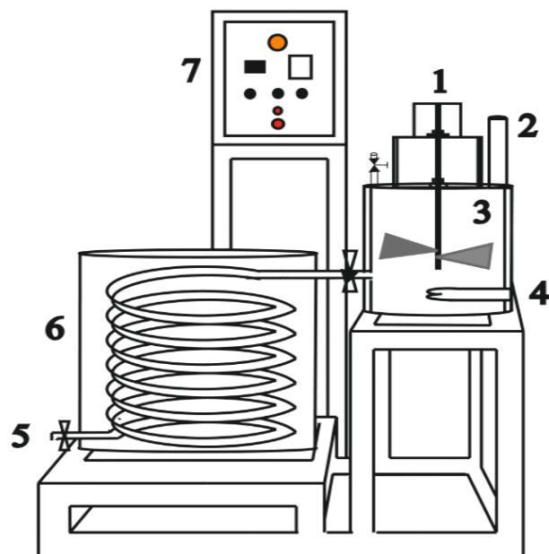
Gambar 1. Dimensi Alat Ekstraktor Hidrotermal
