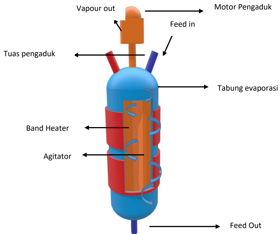
Gambar 8. Dimensi Evaporator
