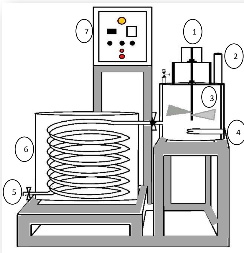
Gambar 2. Dimensi Alat Ekstraktor Hidrothermal
