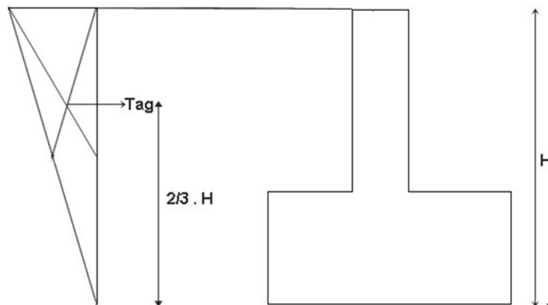
Gambar 2.7 Gaya Tekanan Tanah Akibat Gempa Bumi
