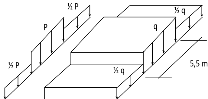
Gambar 2.4 Ketentuan Penggunaan Beban “D”
