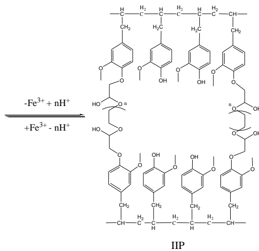
Gambar 3. Sintesis IIP Fe
