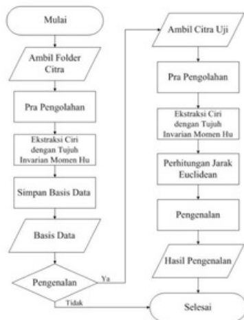
Gambar 1 Diagram AlirPerancanganSistem
