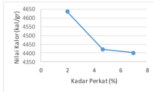
Gambar 3. Hubungan kadar perekat dengan nilai kalor pada komposisi yang sama
