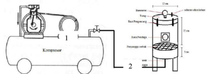
Gambar 1. Rangkaian Alat Penelitian
