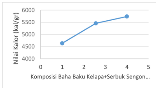
Gambar 2. Hubungan Komposisi dengan nilai kalor pada prosentase perekat yang sama
