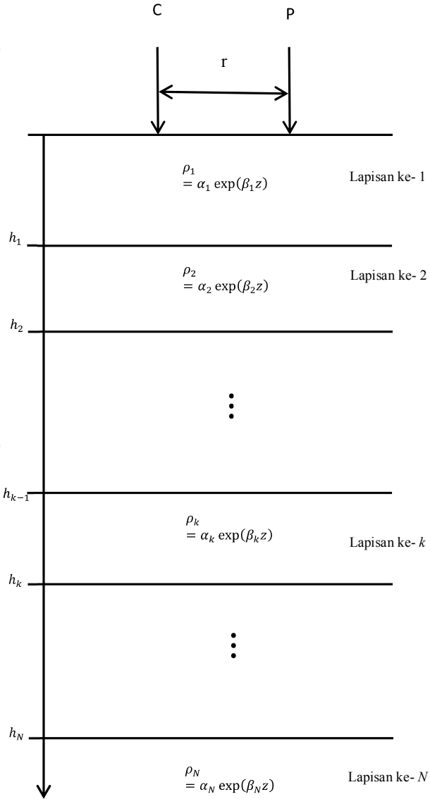
Gambar 1. Ilustrasi Geometri Model Masalah Potensial Listrik Pada Permukaan Bumi
