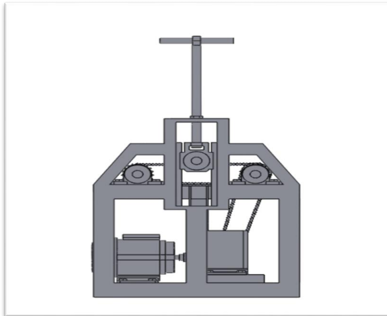
Gambar 2. 1 Desain mesin pengerol pipa
