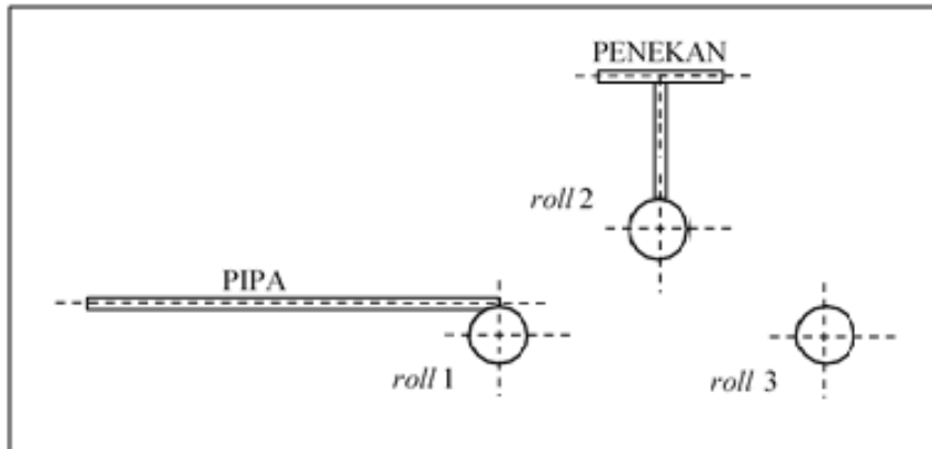
Gambar 2. 2 Posisi awal mulai pengerolan
