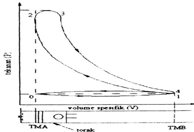
Gambar 2.2 Diagram P-V sebenarnya Mesin Diesel 4 Tak
