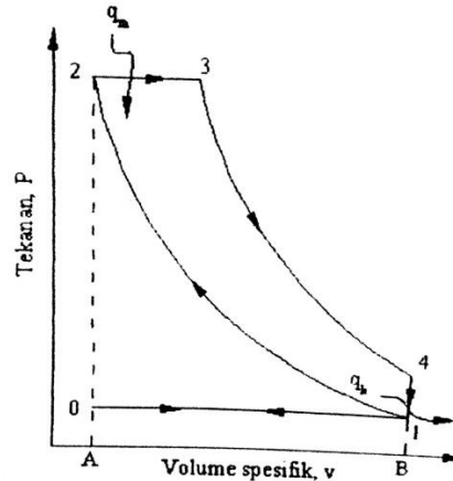
Gambar 2.1 Diagram P-V Teoritis Mesin Diesel 4 Tak
