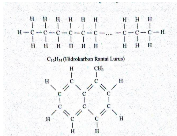
Gambar 2.5 C_{16}H_{34} (Hidrokarbon Rantai Lurus) dan \alpha -Methilnaphthalene
