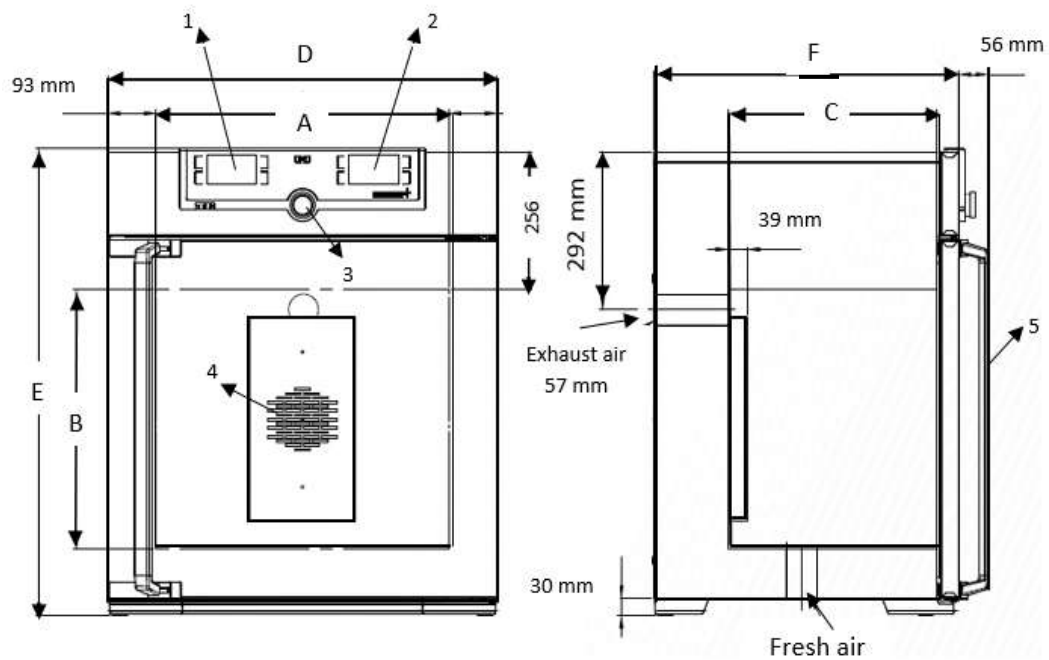
Gambar 3. Dimensi Oven
