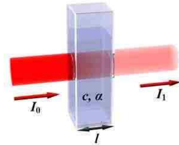
Gambar 4. Proses Penyerapan Cahaya (Setyawan Gadi, 2015)
