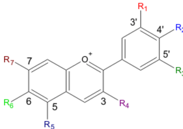
Gambar 2. Struktur Kimia Senyawa Antosianin
