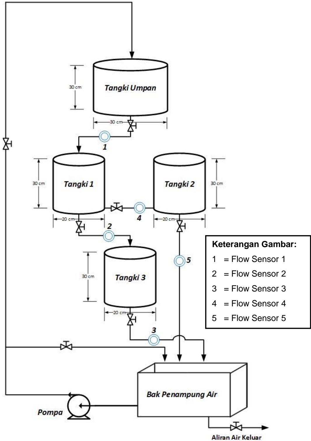
Gambar 24. Skema Alat Dinamika Proses
