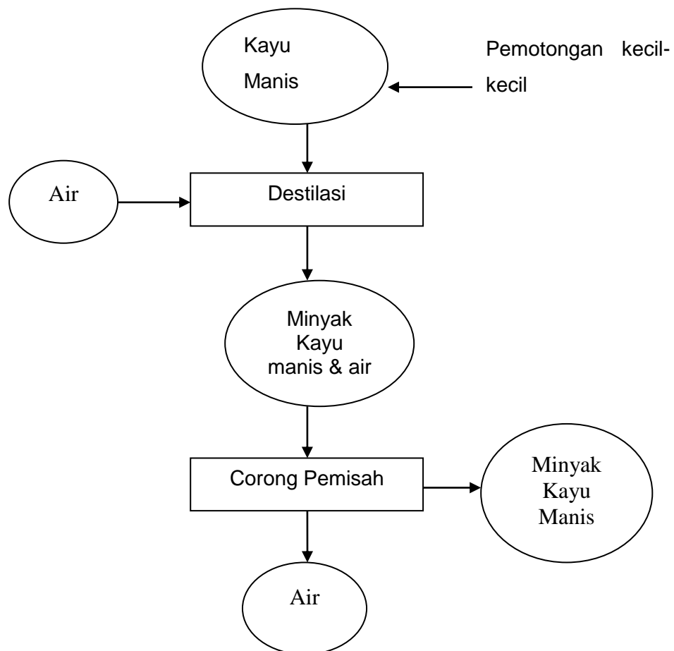
Gambar 2. Diagram Alir Pembuatan Minyak Kayu Manis
