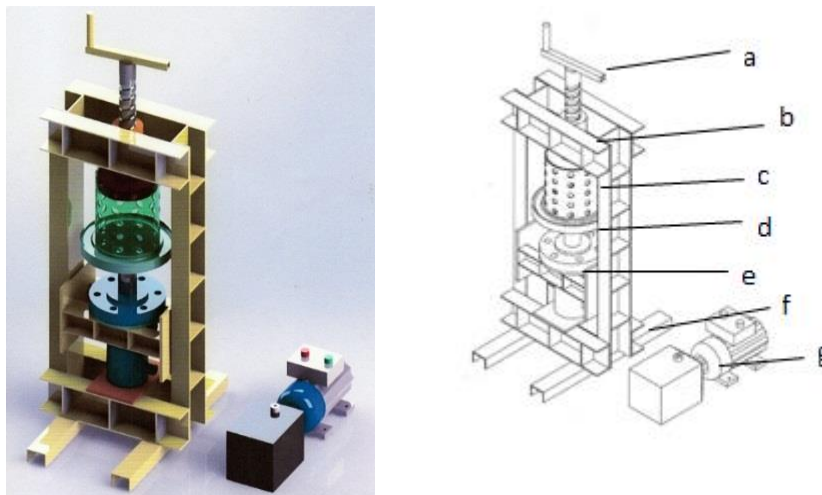
Gambar 5. Alat Press Hidrolik
