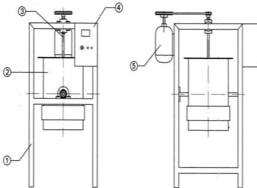
Gambar 4. Rangkaian Alat Digester
