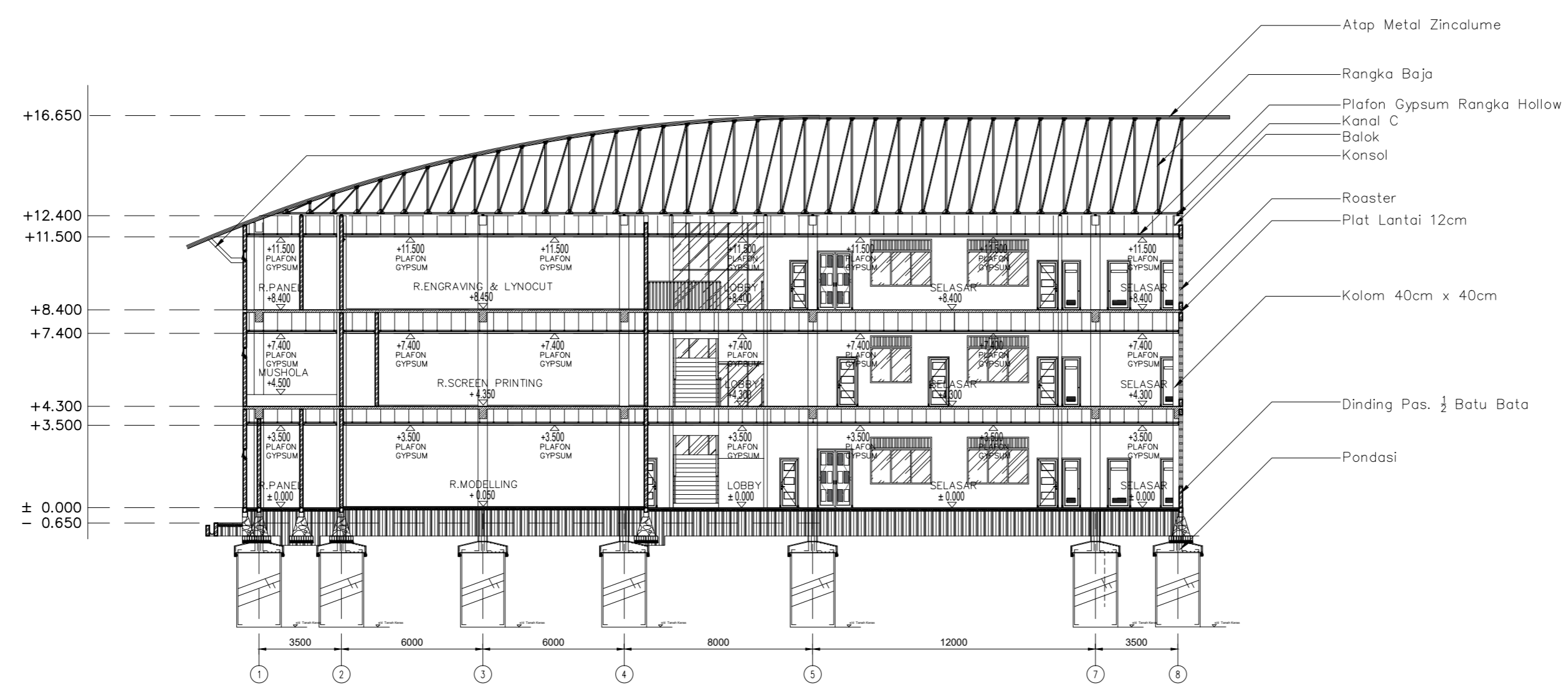
POTONGAN A-A
