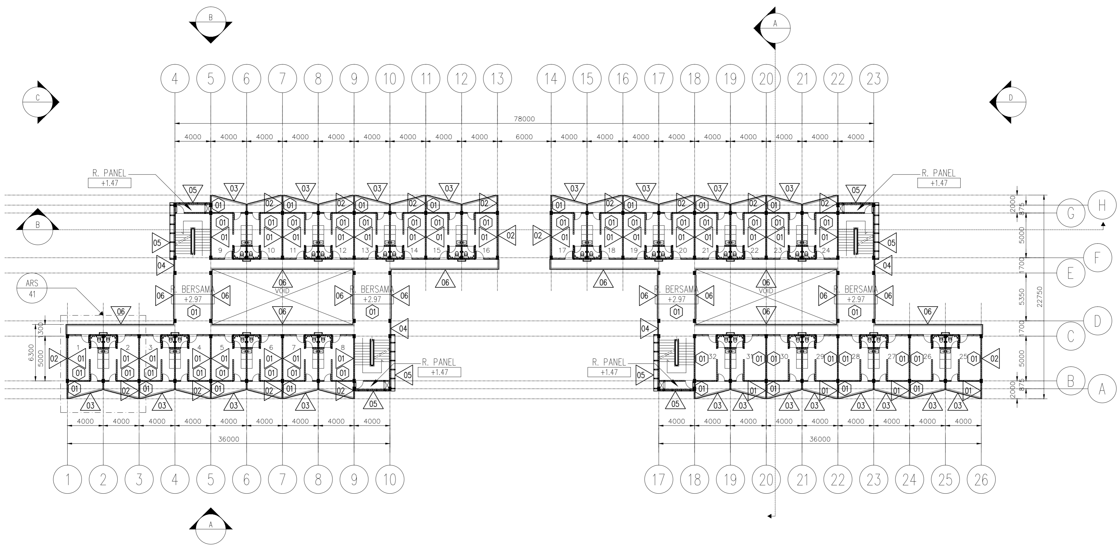
ARS DENAH LANTAI SATU 04 1:250
