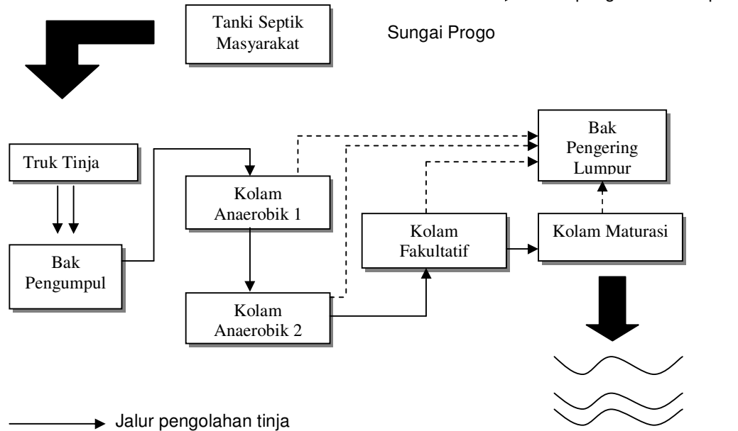
Gambar 1 Diagram Alir Pengoperasian IPLT Kota Magelang
