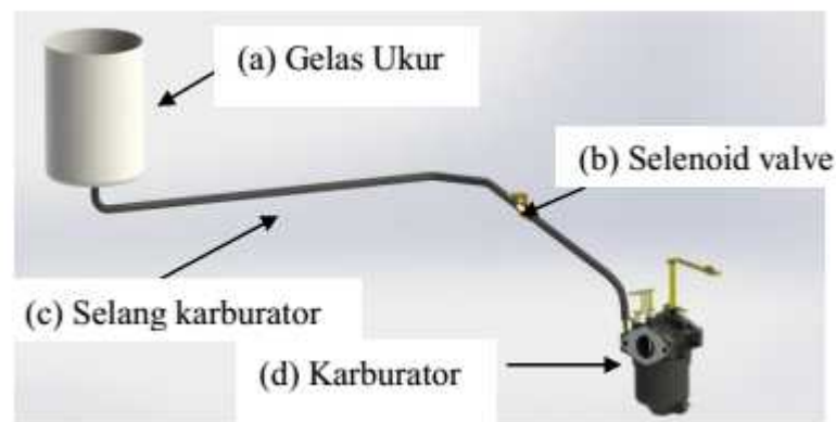
Gambar 2.3 Skema sistem bahan bakar bensin pada genset
