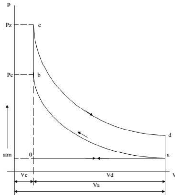
Gambar 2.5 Diagram P-V Teoritis Motor Bensin 4 Langkah.
