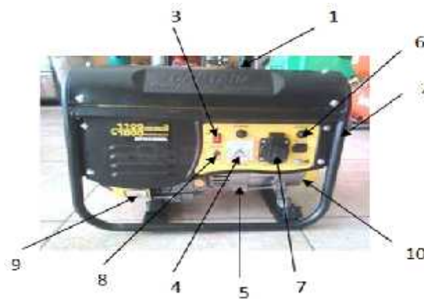
Gambar 2.8 Bagian – bagian Genset
