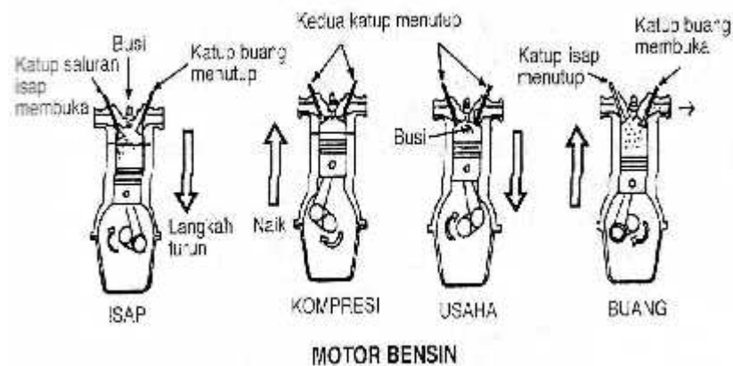
Gambar 2.1 Cara kerja motor bensin 4 langkah
