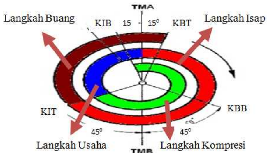
Gambar 2.2 Diagram katup isap dan katup buang
