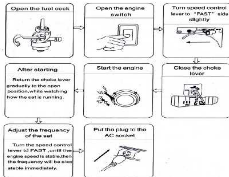
Gambar 2.9 Prosedur start pada mesin genset
