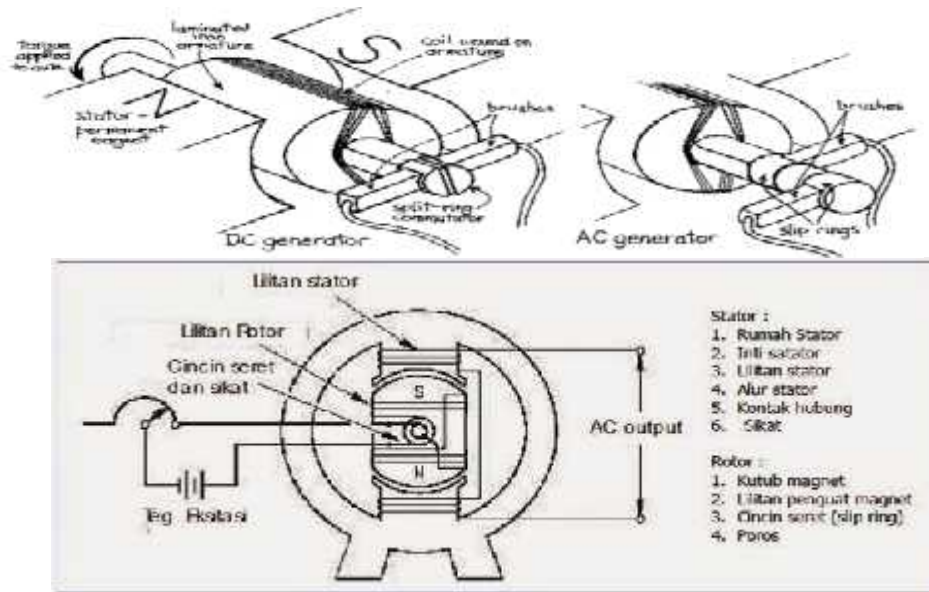
Gambar 2.7 Prinsip kerja mesin genset
