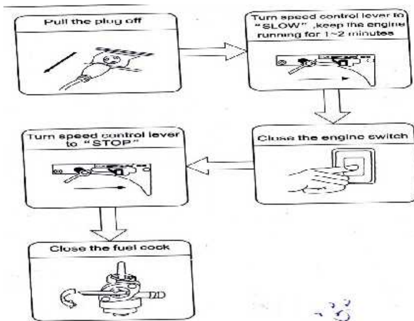
Gambar 2.10 Prosedur mematikan mesin genset
