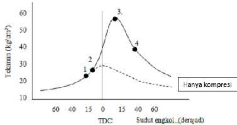
Gambar 2.6 Grafik Pembakaran Sempurna Motor Bensin
