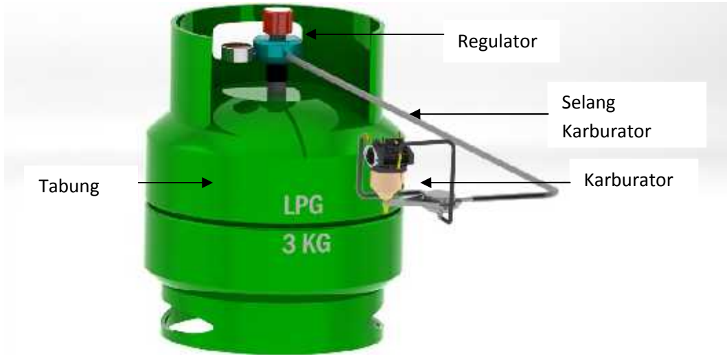
Gambar 2.3 skema sistem bahan bakar LPG pada genset
