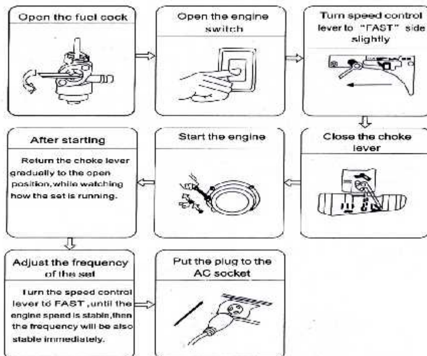
Gambar 2.7 Prosedur start pada mesin genset 1100 Watt
