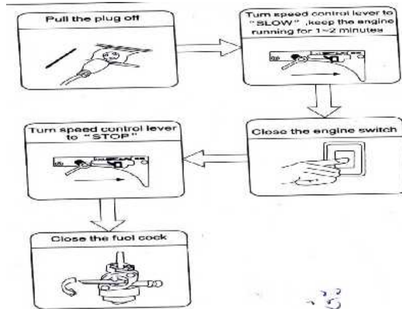
Gambar 2.8 Prosedur mematikan mesin genset
