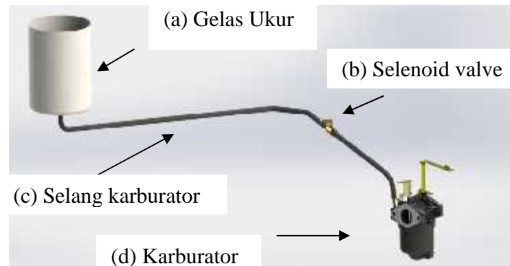
Gambar 2.2 skema sistem bahan bakar bensin pada genset
