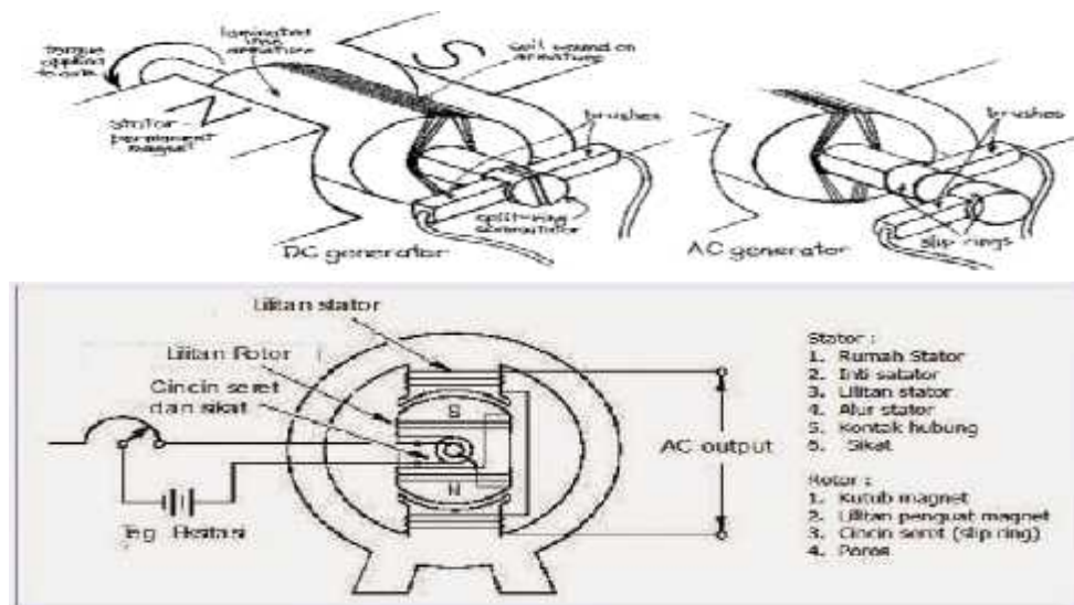
Gambar 2.5 Prinsip kerja mesin genset
