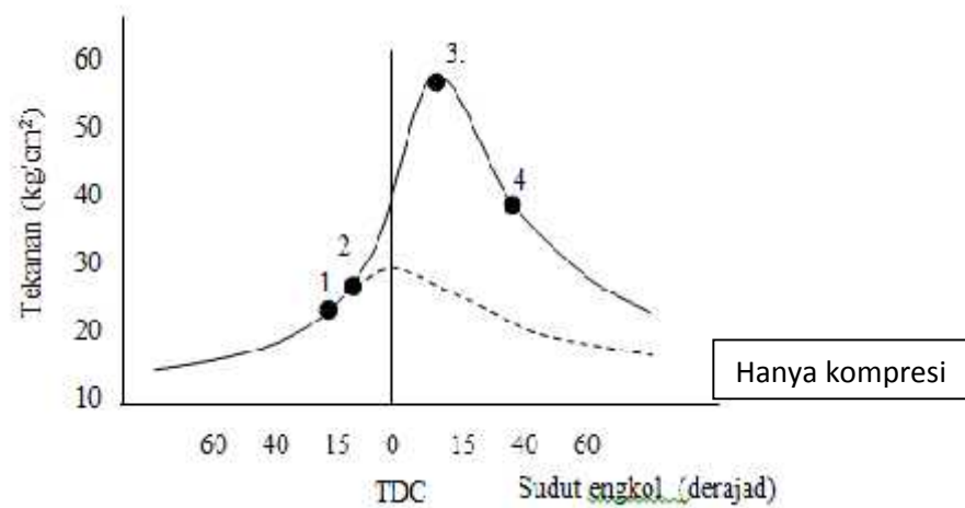
Gambar 2.4 Grafik pembakaran sempurna motor bensin
