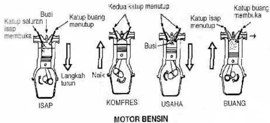
Gambar 2.1 Cara kerja motor bensin 4 langkah
