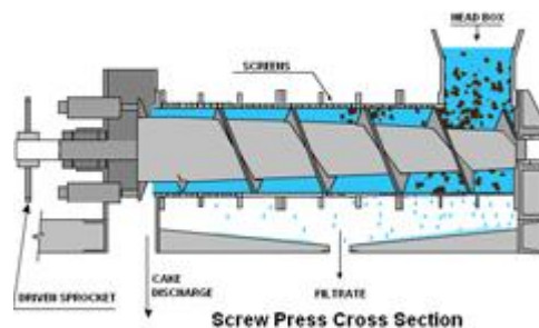
Gambar 4. Alat Pengepres Ulir
