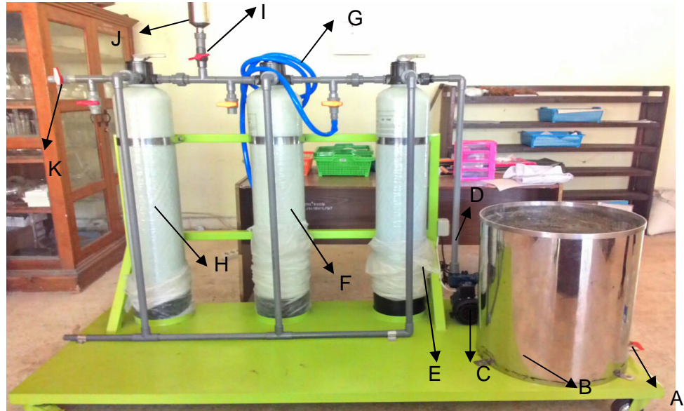
Gambar 2. Alat Ion Exchanger Resin Anion Kation dan Karbon Aktif
