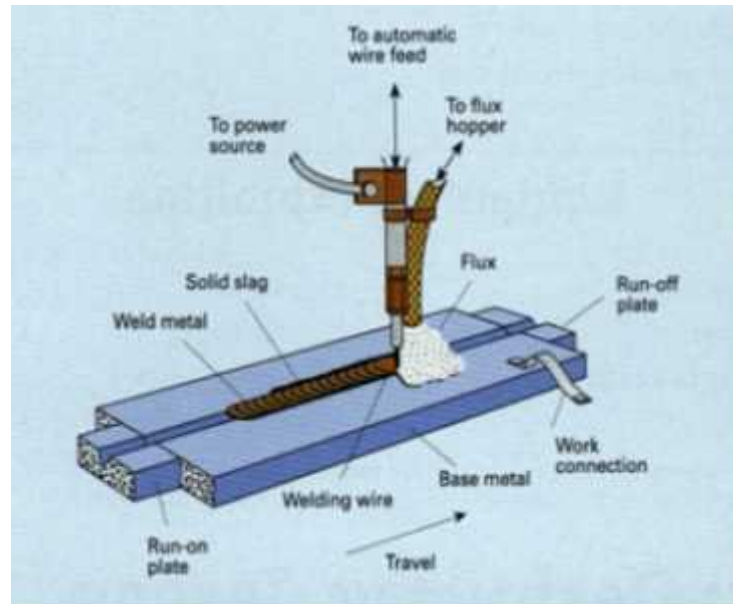
Gambar 2.4 Las Busur Rendam
