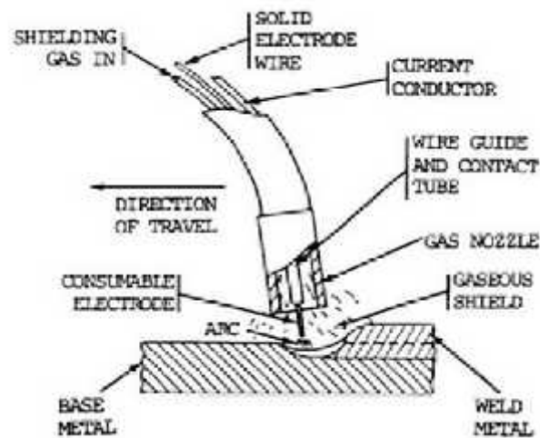
Gambar 2.3 Las MIG
