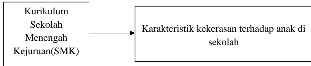
Gambar 2. Kerangka konsep
