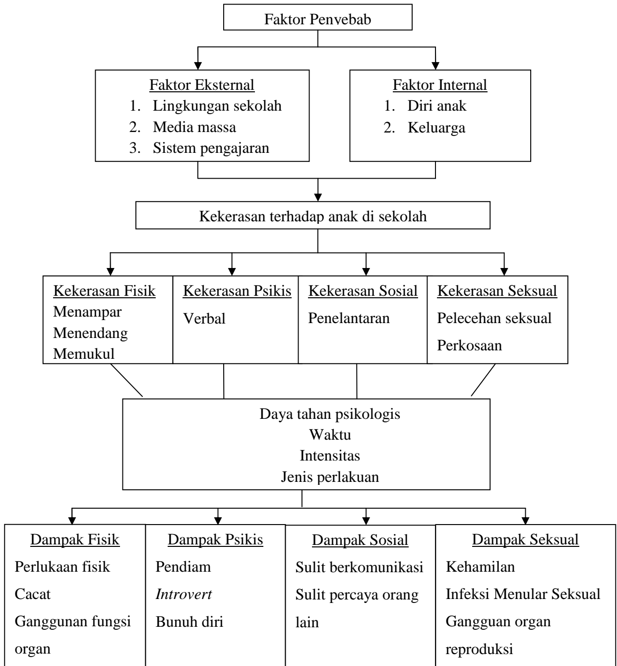
Gambar 1. Kerangka teori
