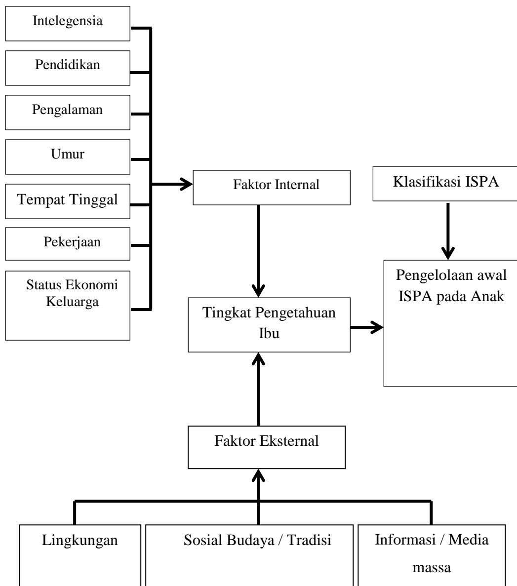
Gambar 1. Kerangka teori
