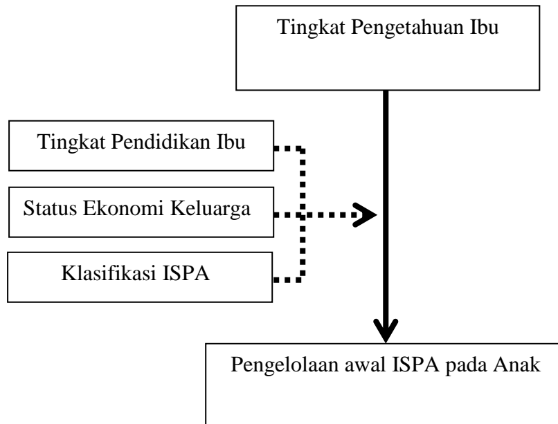
Gambar 2. Kerangka konsep
