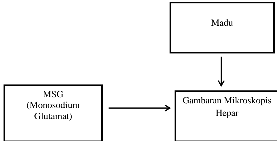
Gambar 4. Kerangka Konsep
