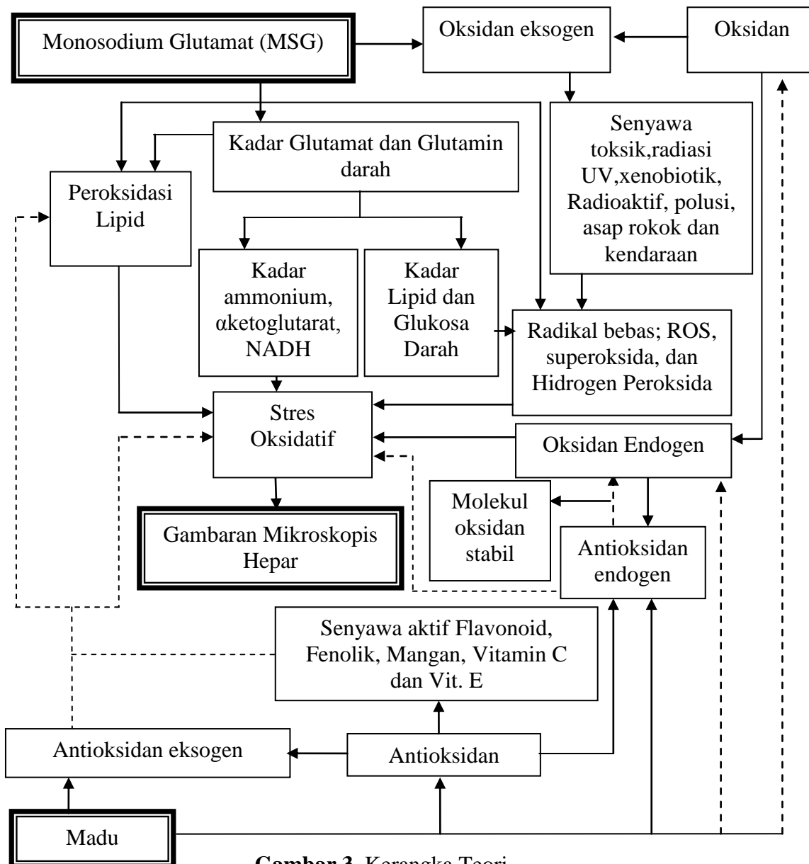
Gambar 3. Kerangka Teori
