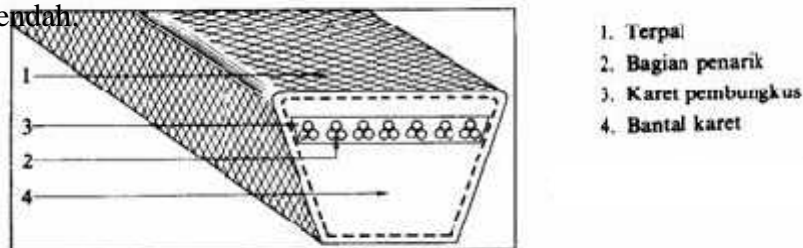
Gambar 2.2 Konstruksi V-Belt
