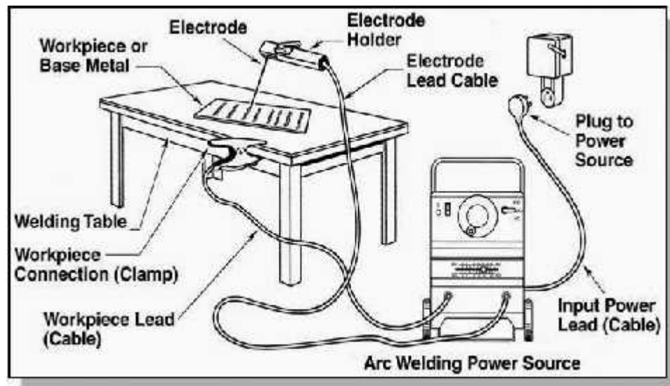
Gambar 2. 5 Rangkaian Proses Pengelasan SMAW
