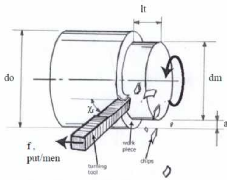
Gambar 2. 9 Skema Proses Bubut
