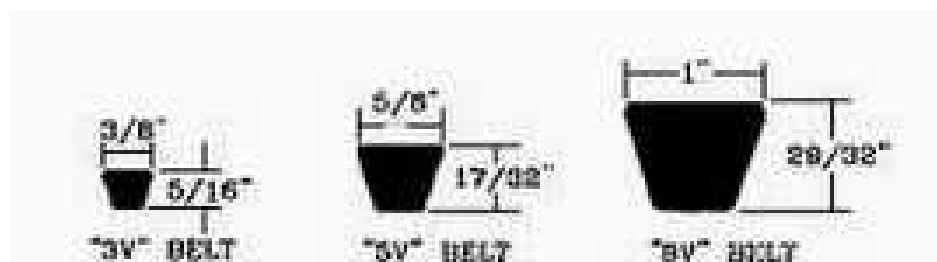
Gambar 2. 3 V-Belt Konvensional Tipe Sempit
