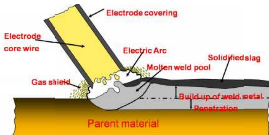
Gambar 2. 6 Prinsip Dasar Pengelasan SMAW
