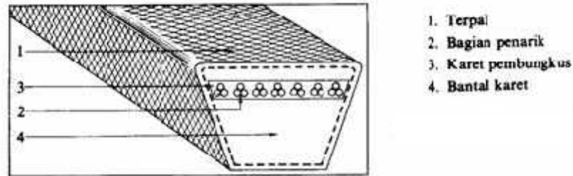
Gambar 2. 1 Konstruksi V-Belt
