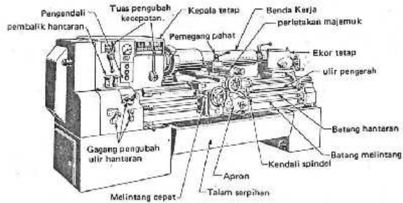
Gambar 2. 8 Gambar skematis Mesin Bubut dan nama bagian-bagiannya
