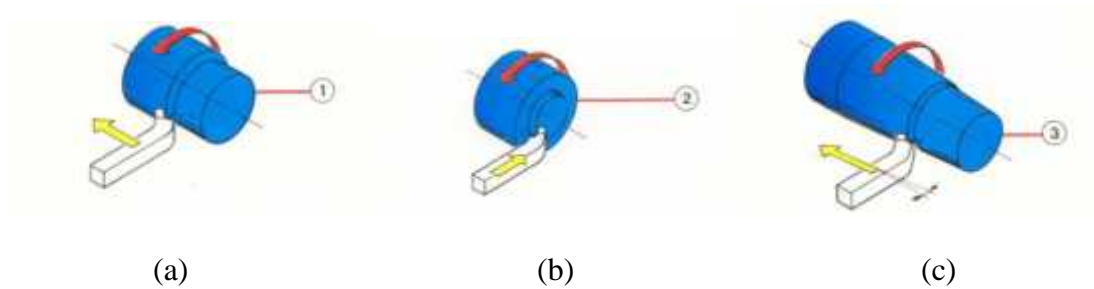
Gambar 2. 7 Proses bubut rata, bubut permukaan, dan bubut tirus
