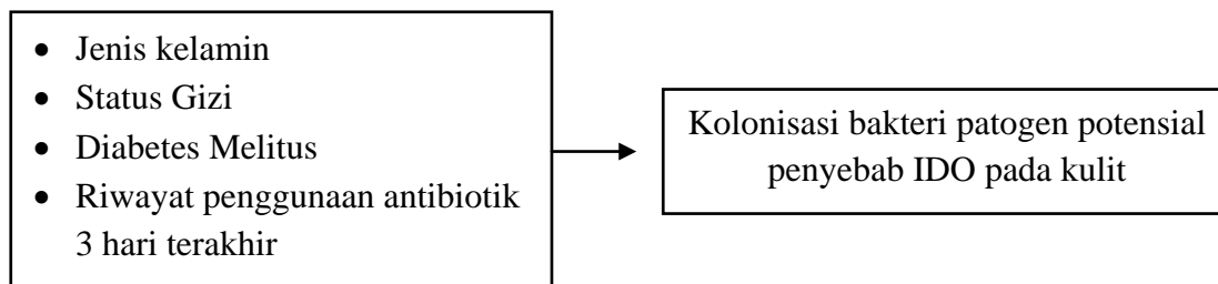
Gambar 24. Kerangka konsep.
