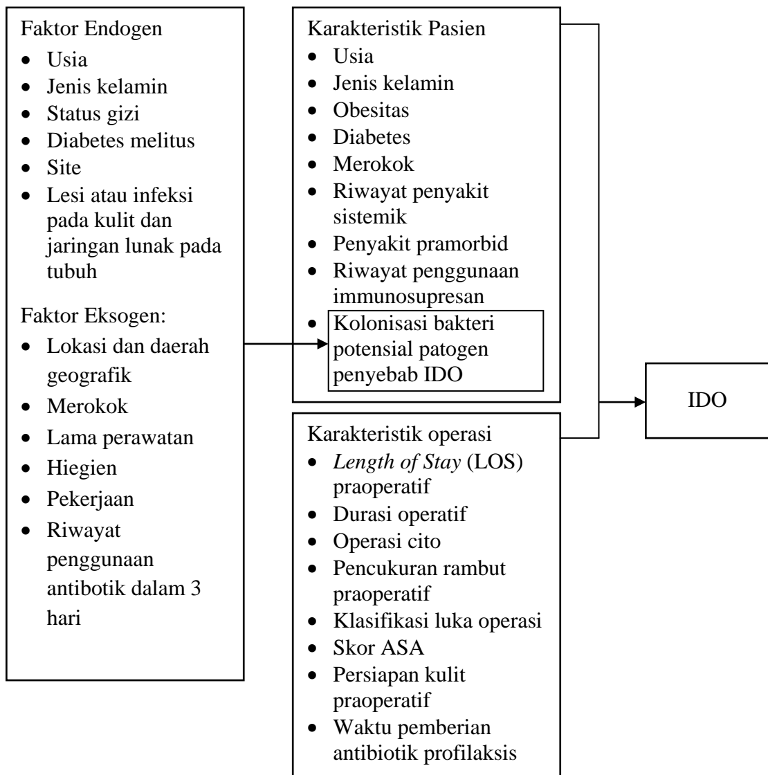
Gambar 23. Kerangka teori.
