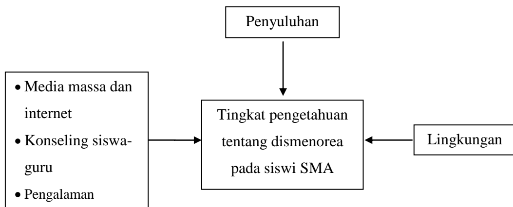
Gambar 3. Kerangka konsep
