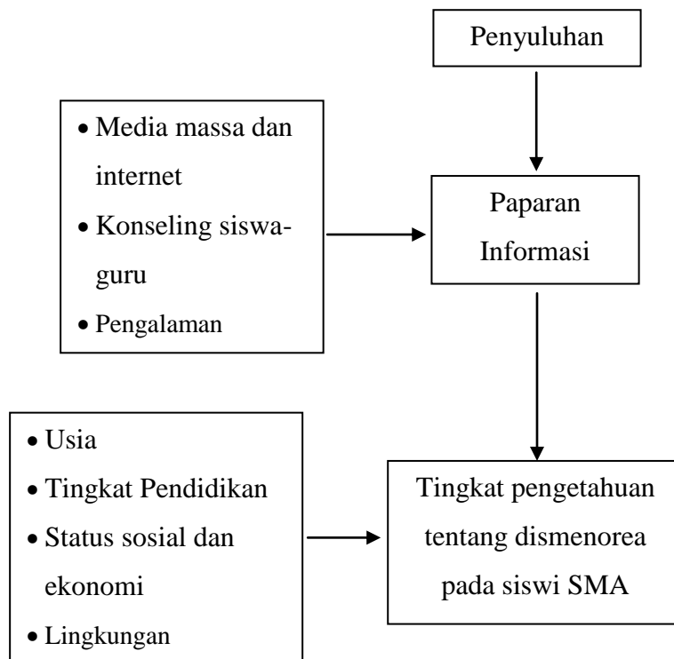
Gambar 2. Kerangka teori
