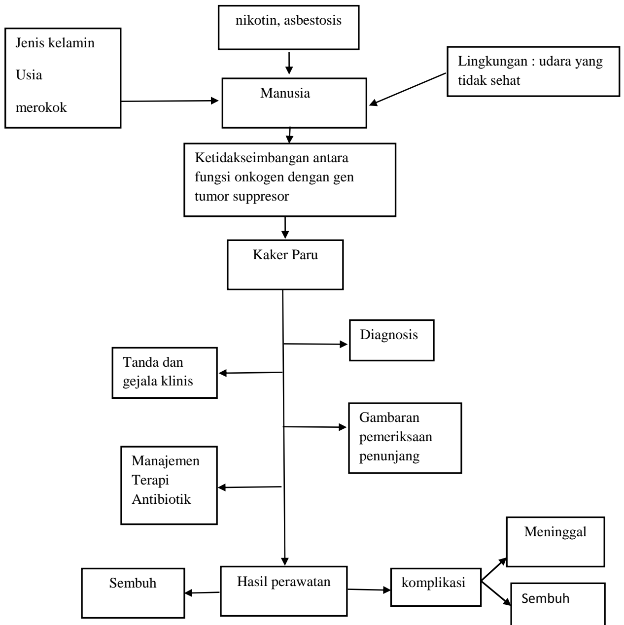
Gambar 1. Kerangka Teori
