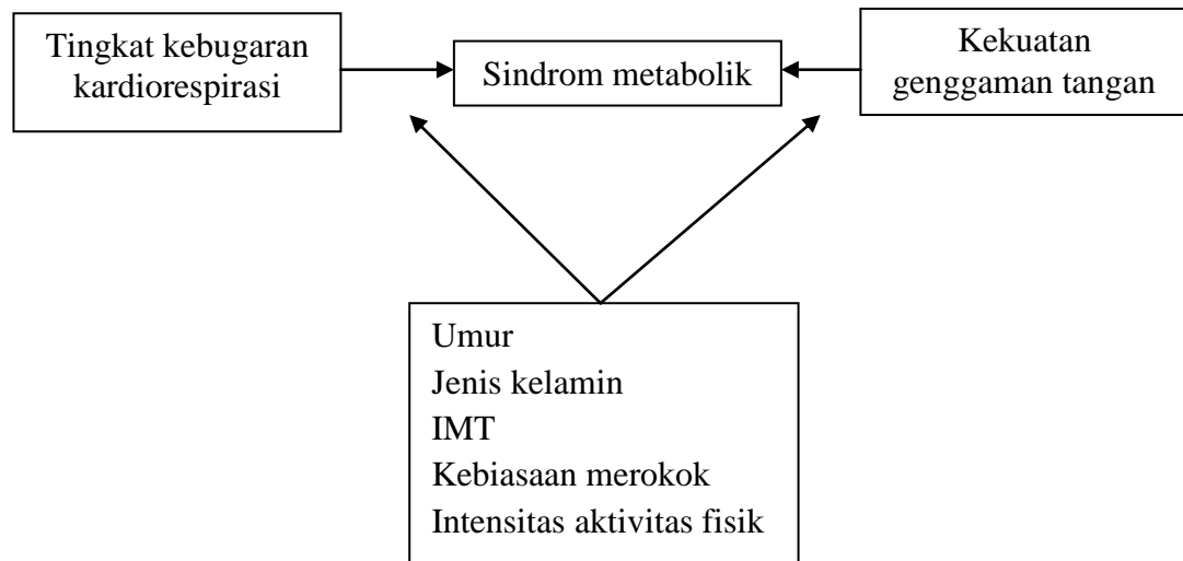
Gambar 5. Kerangka konsep
