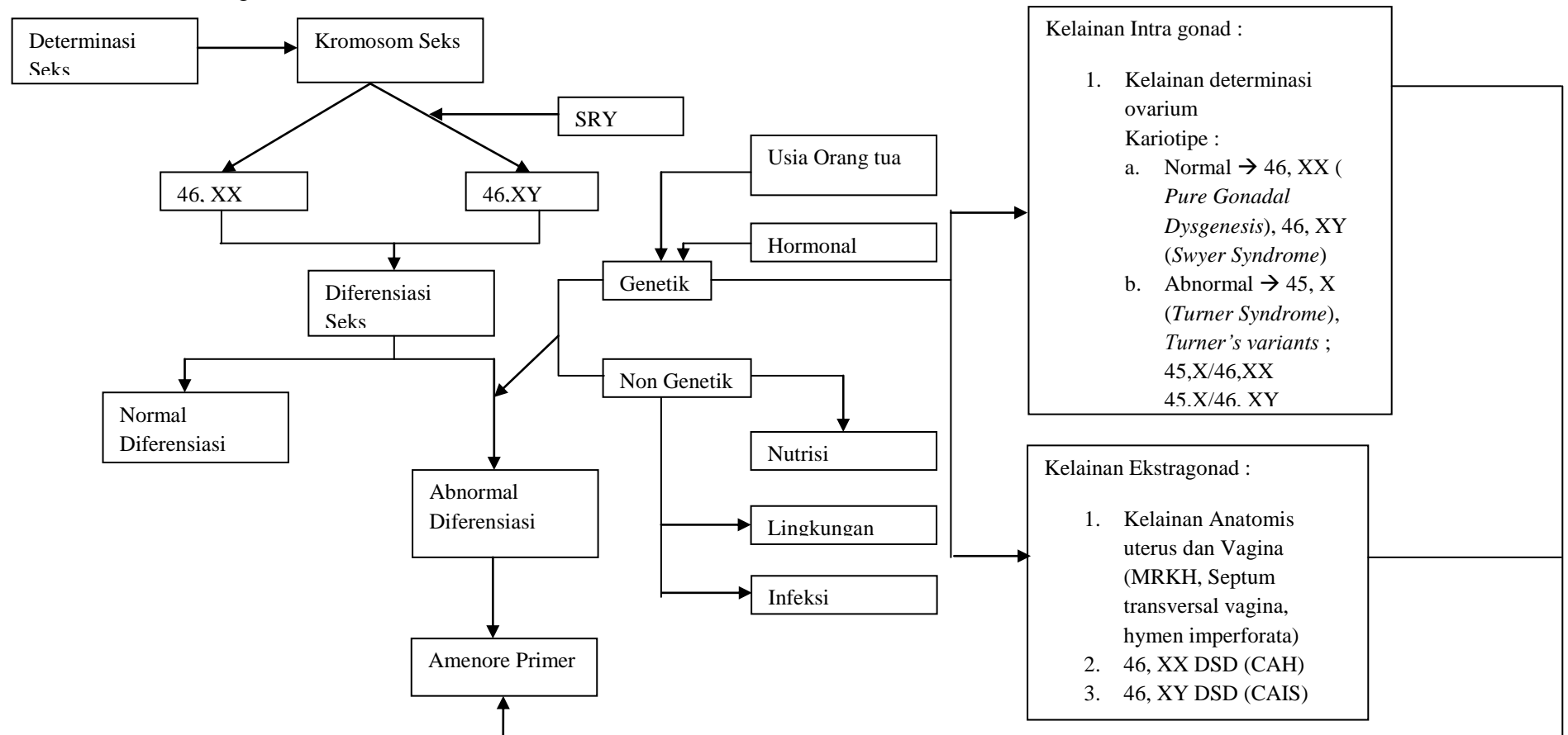
Gambar 5. Kerangka Teori
