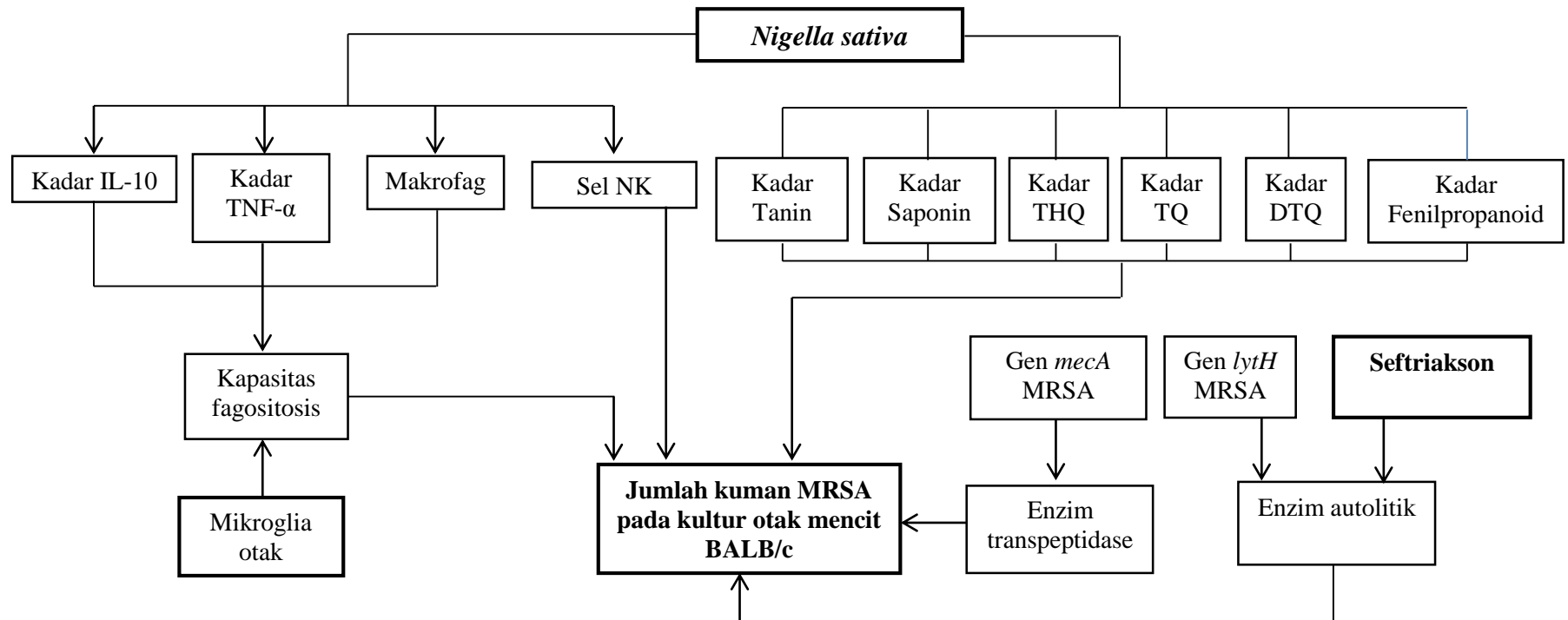
Gambar 3. Kerangka teori
