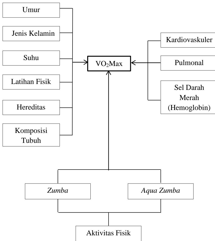
Gambar 9. Kerangka teori
