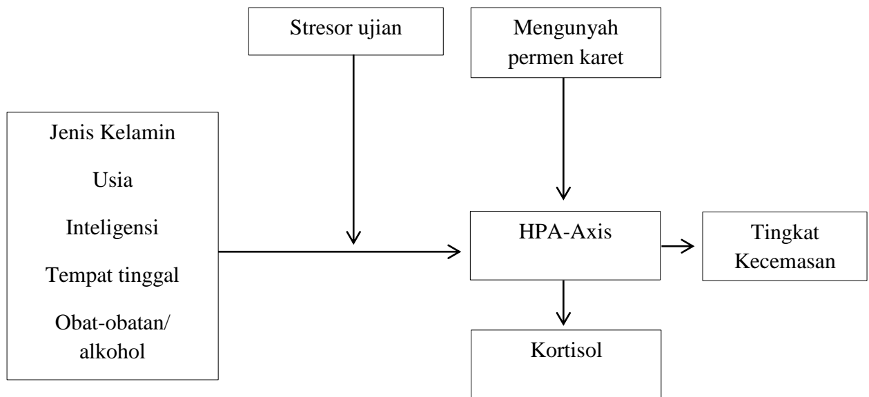
Gambar 1. Kerangka teori
