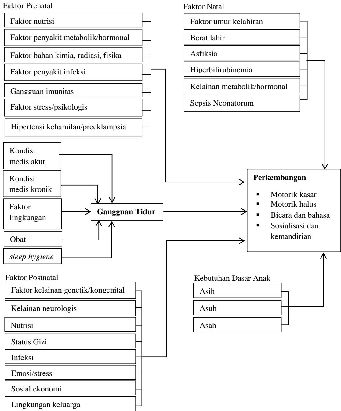
Gambar 1. Kerangka teori
