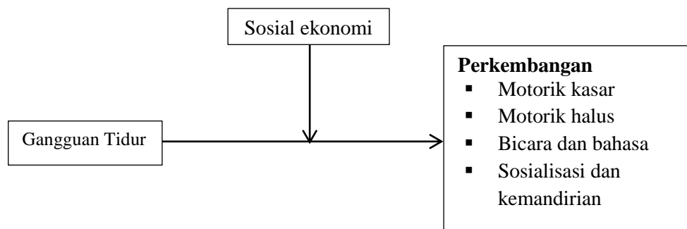
Gambar 2. Kerangka konsep
