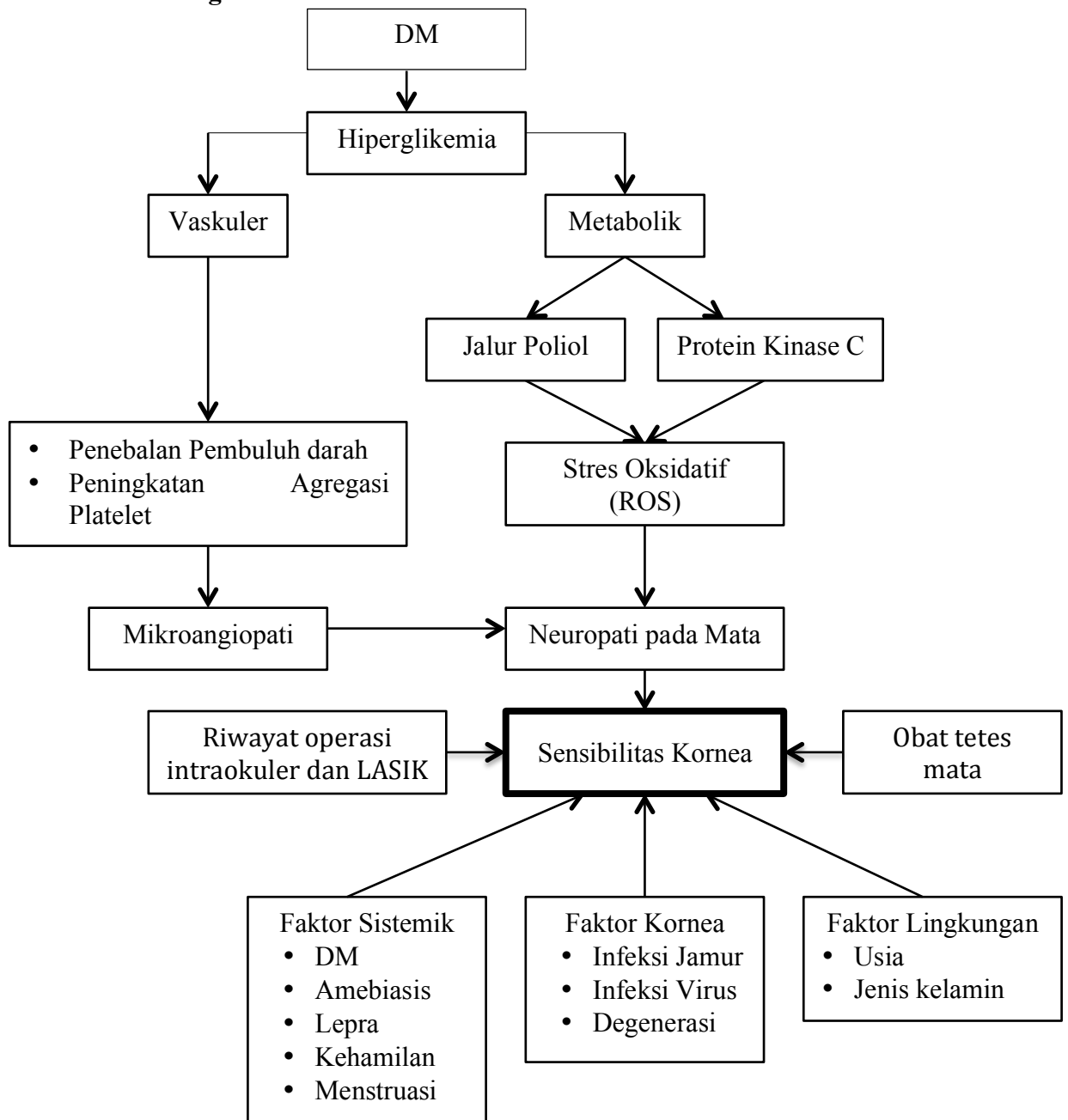
Gambar 4. Kerangka Teori
