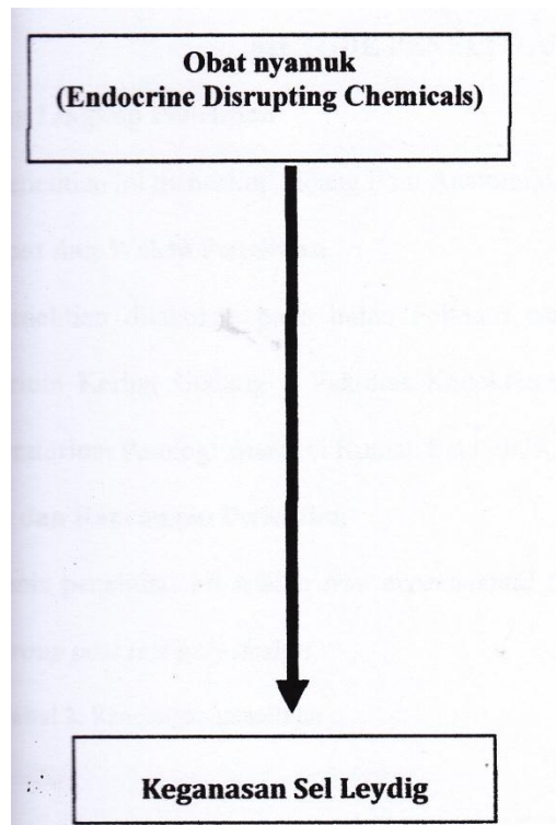
Gambar 9 : Kerangka Konsep
