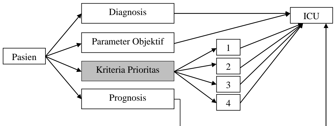
Gambar 1. Kerangka Teori
