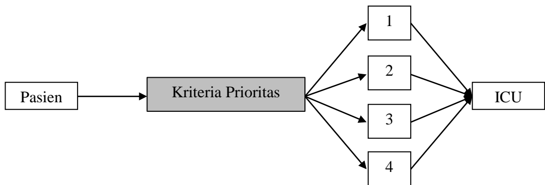
Gambar 2. Kerangka Konsep
