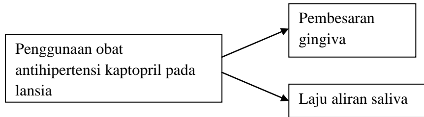
Gambar 6. Kerangka Konsep
