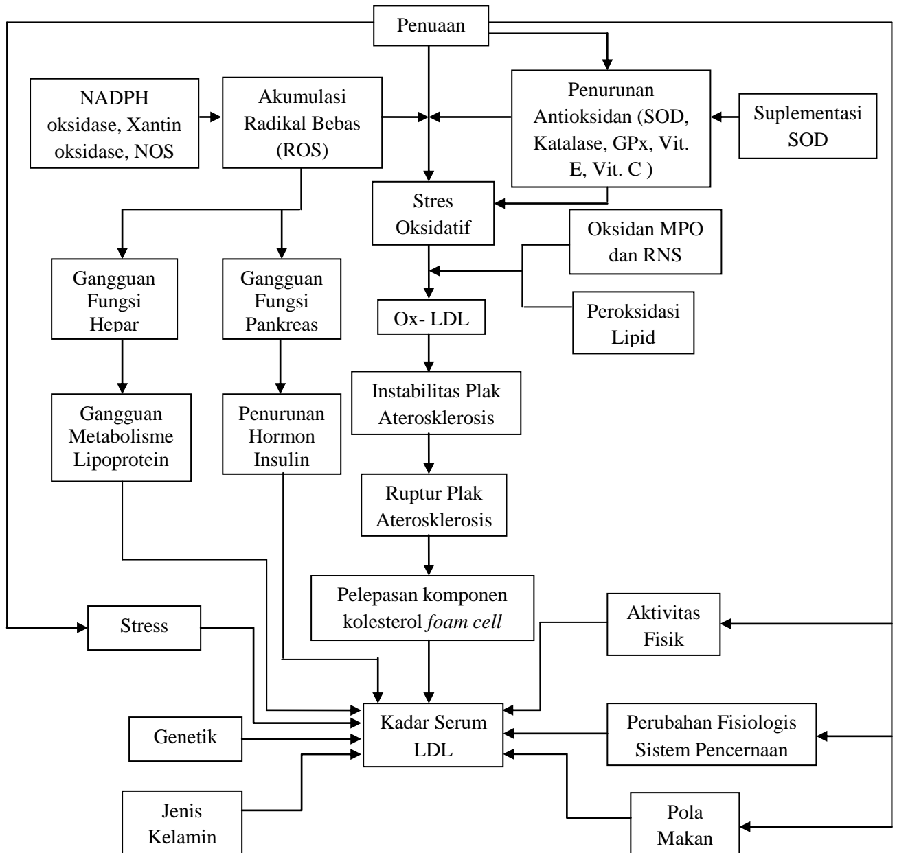
Gambar 8. Kerangka Teori
