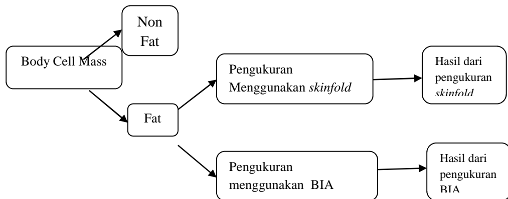
Gambar 1. Kerangka Teori
