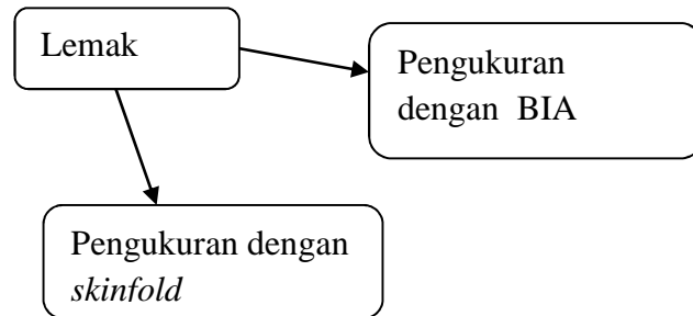
Gambar 2. Kerangka Konsep
