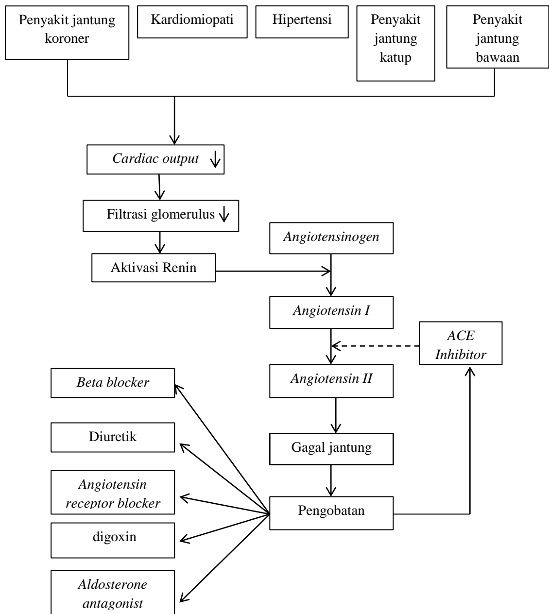
Gambar 2. Kerangka Teori
