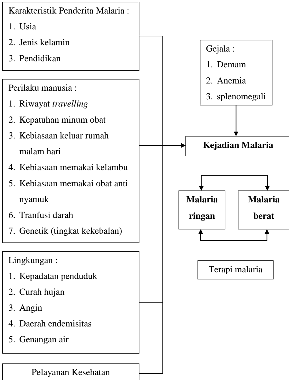
Gambar 6. Kerangka Teori
