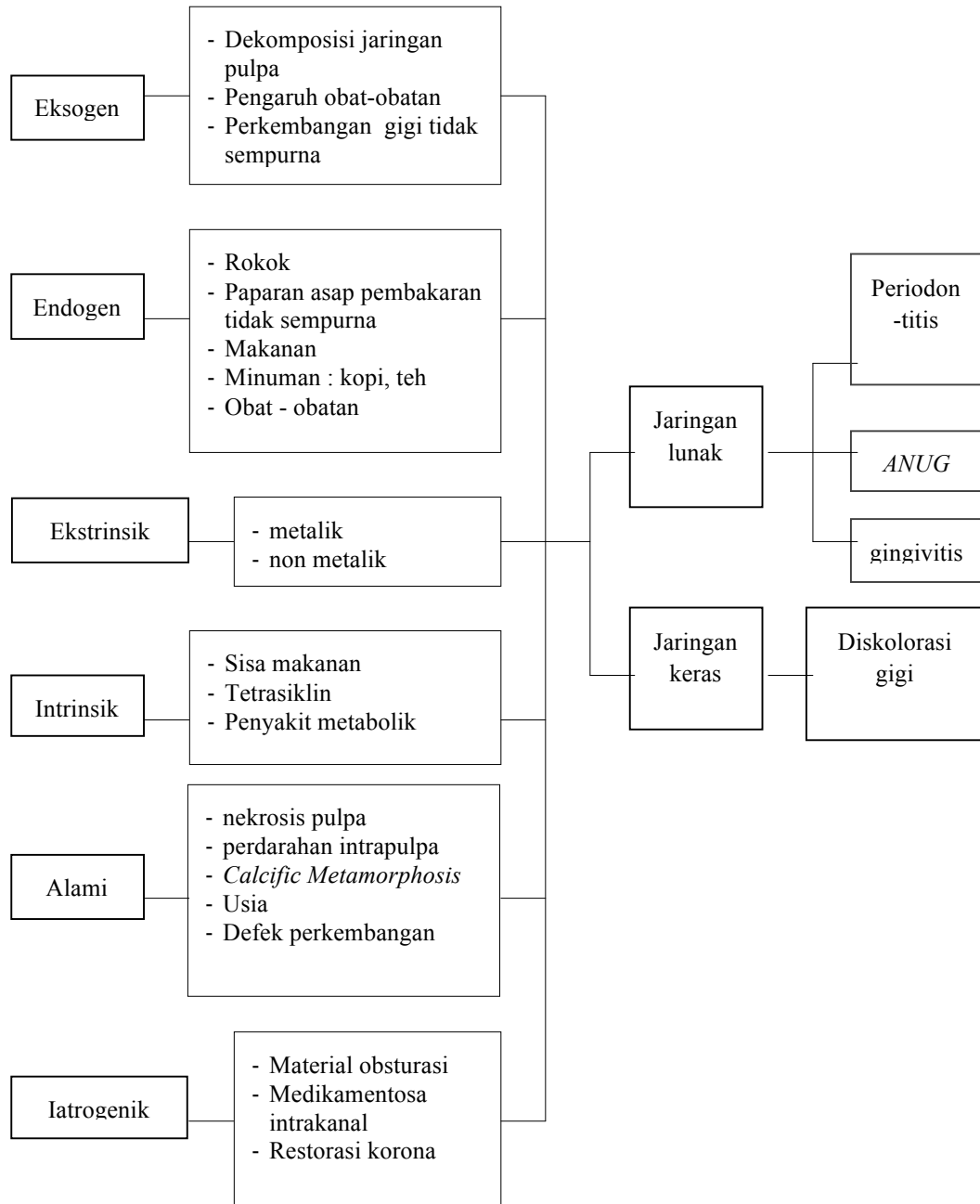
Gambar 6. Kerangka teori
