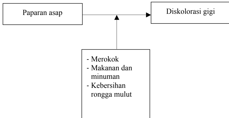
Gambar 7. Kerangka konsep
