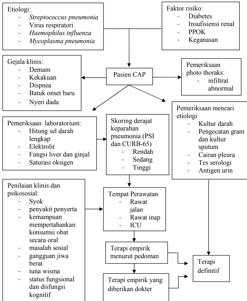
Gambar 3. Kerangka teori
