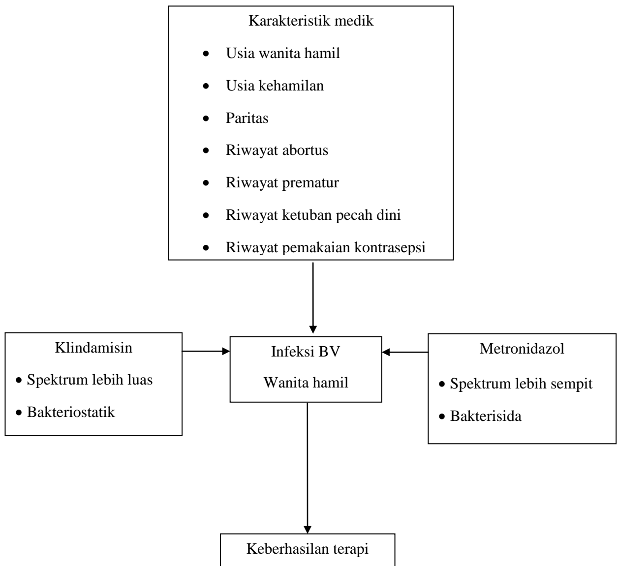
Gambar 4. Kerangka Teori
