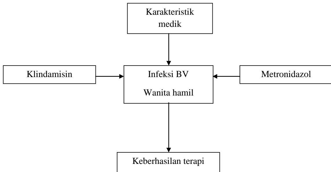
Gambar 5. Kerangka konsep
